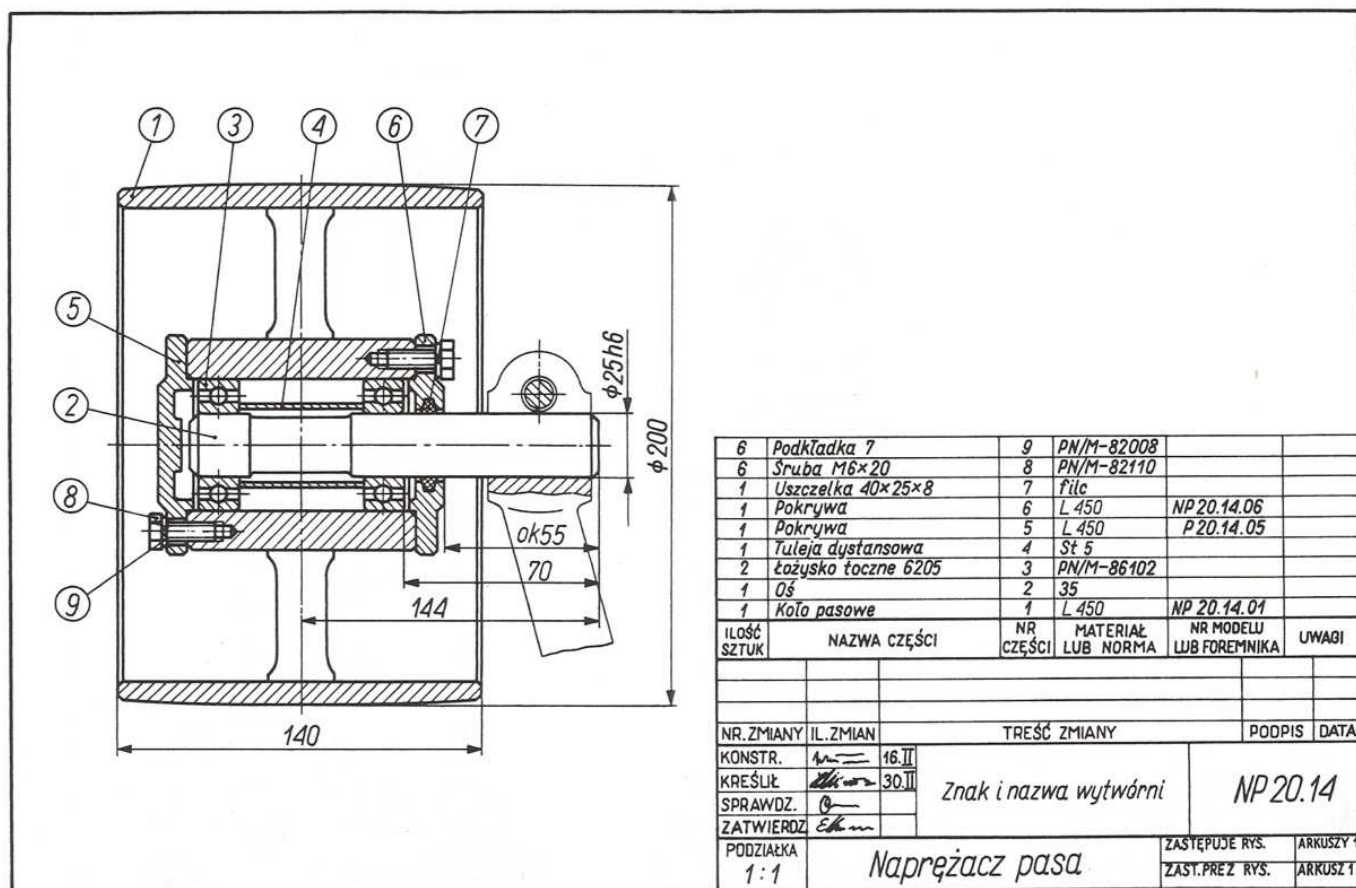
Rys. 4. Rysunek złożeniowy naprężacza pasa (przykład)
