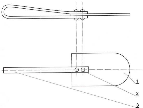
Rys. 2. Rysunek złożeniowy łopatk
