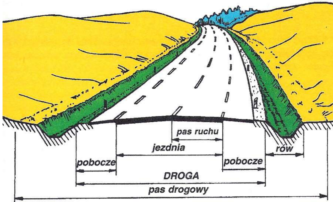
Droga z wyznaczonymi pasami ruchu
